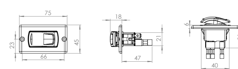
Interrupteur Comfort
